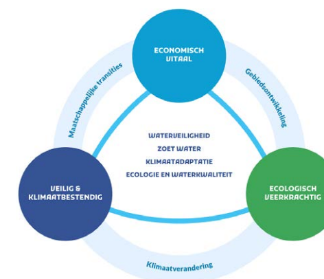
De basis (de driehoek) van de Zuidwestelijke Delta
