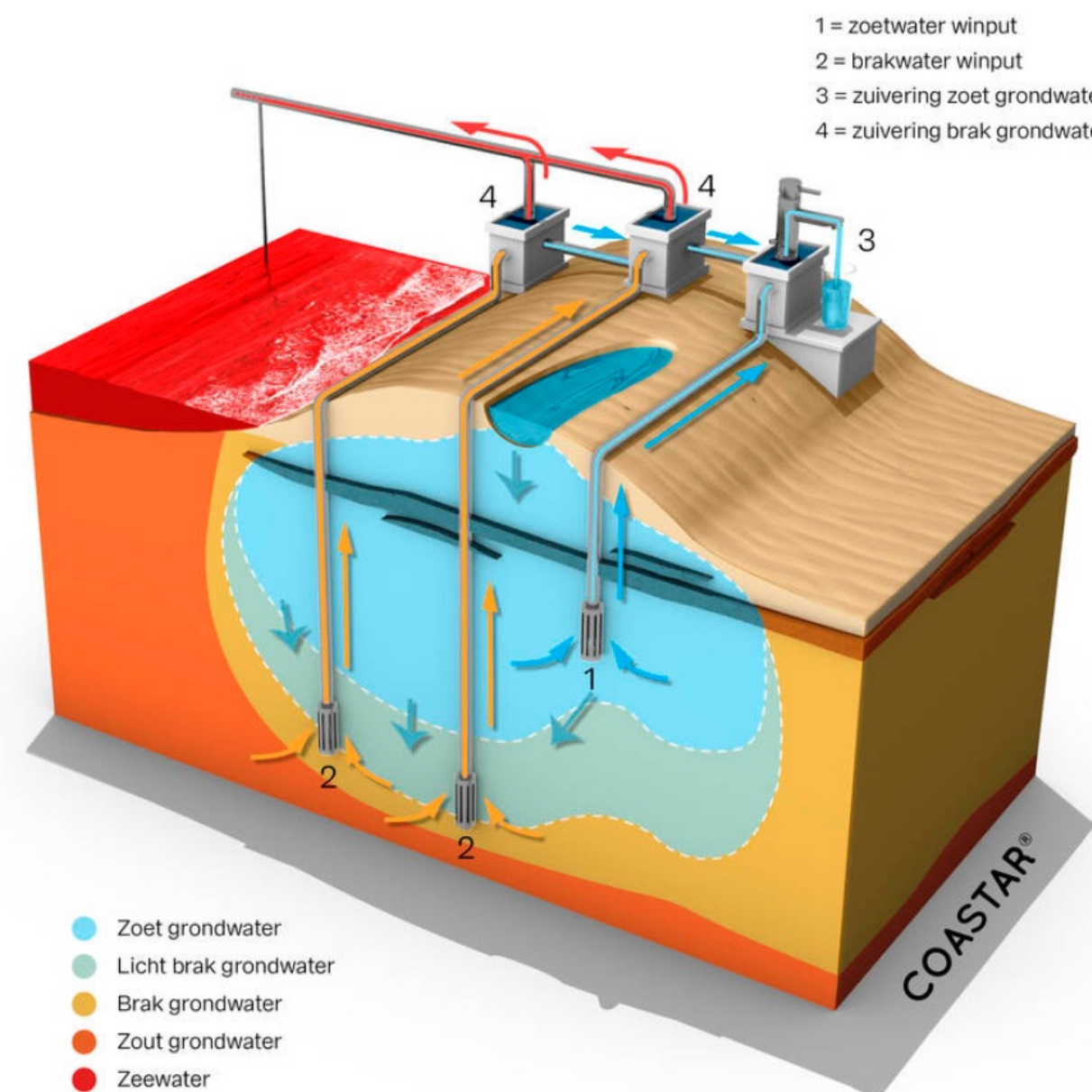
Schematische voorstelling
