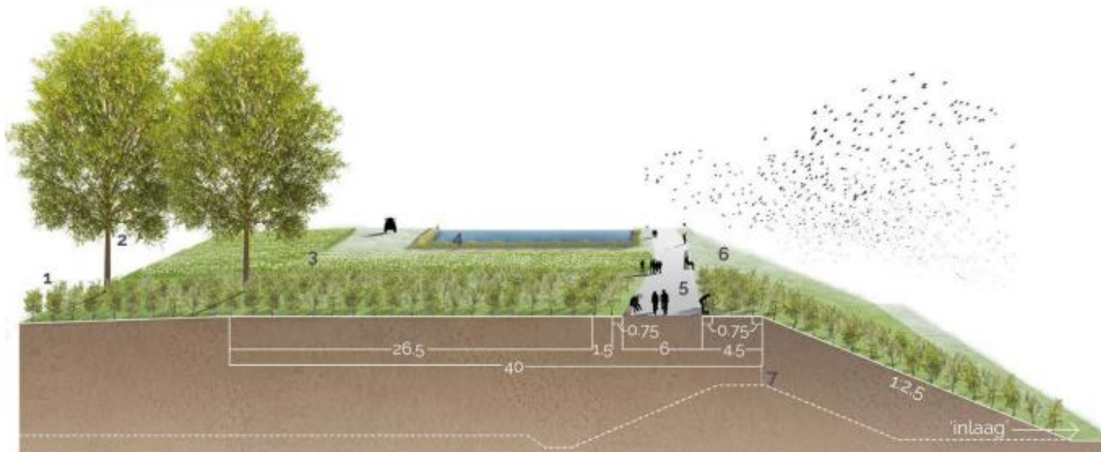
Detail dijkkruin
