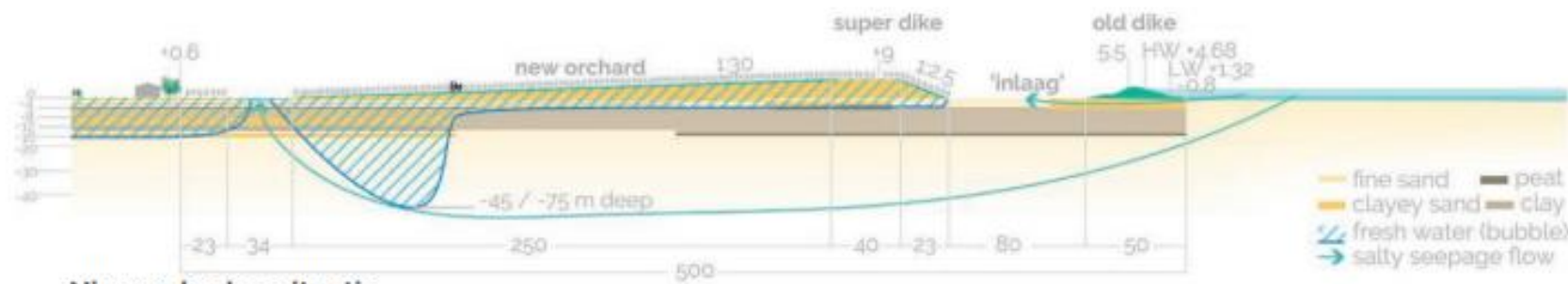
Nieuwe bodemsituatie
