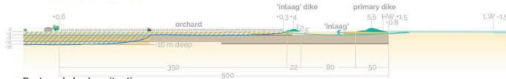
Bestaande bodemsituatie
